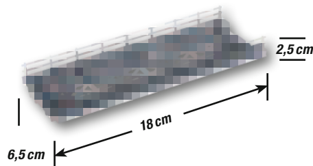
H0 21340 Brückenfahrbahn, gerade Bausatz, steckbar
