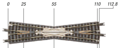
7297020 (R020) Kreuzung 13° , 112,8 mm, mit 2 x Ausgleichsgleis 53,6 mm (1 Stück) - mit Holzschwellen (1 Stück)
