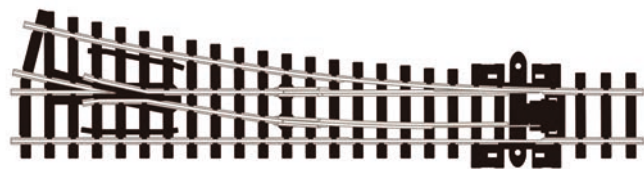
Weiche mittel, L123,7 mm, R457 mm, 12°
