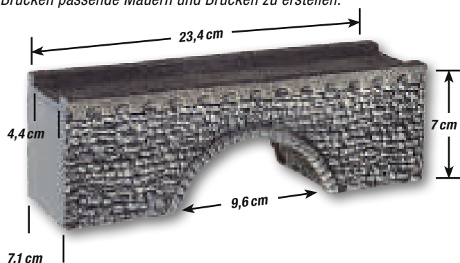
H0 58690 Achtobel-Brücke Brücken-Fertigmodell aus Struktur-Hartschaum
