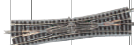
7297058 (R058) Bogenweiche rechts , R220/195-30°, 112,8 mm mit 1 x angeschnittenem, gebogenem Gleis, - mit Betonschwellen (1 Stück)
