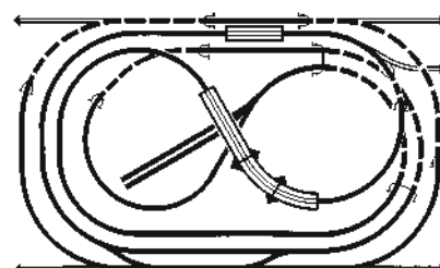
Gleisbild Grundanlage Spur H0
