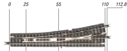
7297039 (R039) Elektr. Weiche links , R490-13°, 110 mm, mit 1 x angeschnittenem geraden Gleis, 110 mm - mit Holzschwellen (1 Stück)
