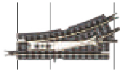
7297022 (R022) Elektr. Weiche links , R127-26°, 55 mm, mit 1 x angeschnittenem geraden Gleis, 55 mm - mit Holzschwellen (1 Stück)
