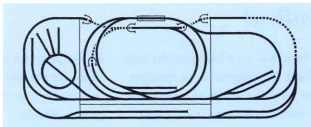
Gleisbild Grundanlage Spur HO + Anbauteile
